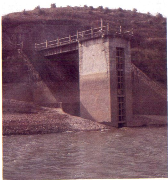
西干渠渠首闸门
