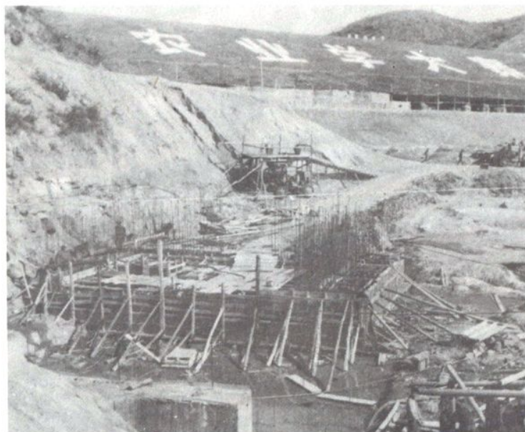
电站厂房基础浇灌
