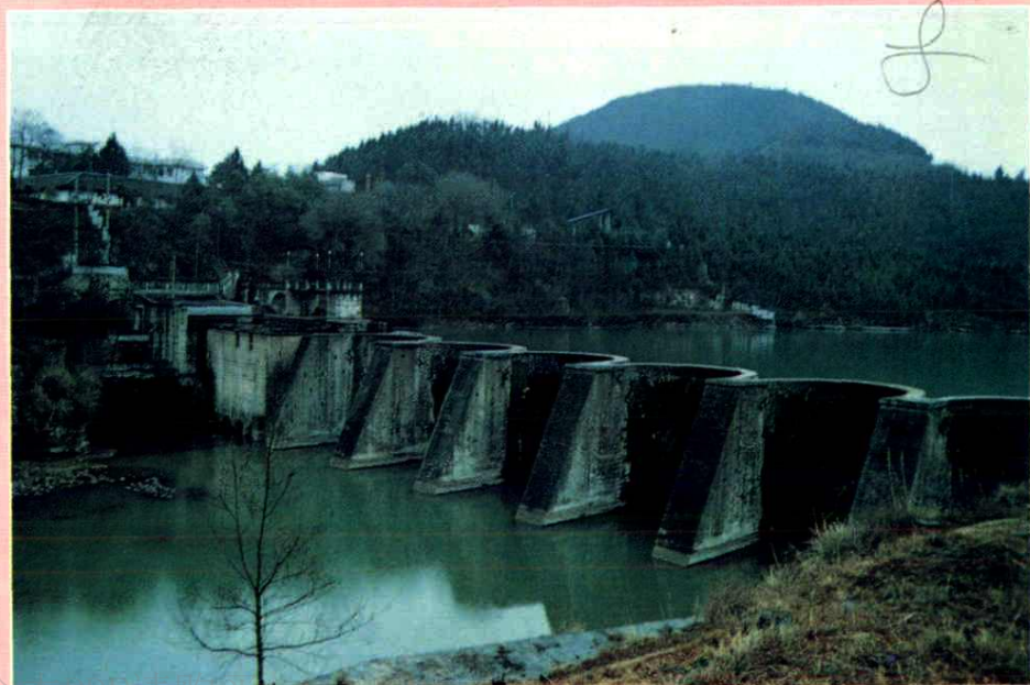
▶红旗堰水库反拱坝全景。
