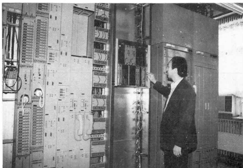
1991 年投入运行的先进通信 设备——光端机
