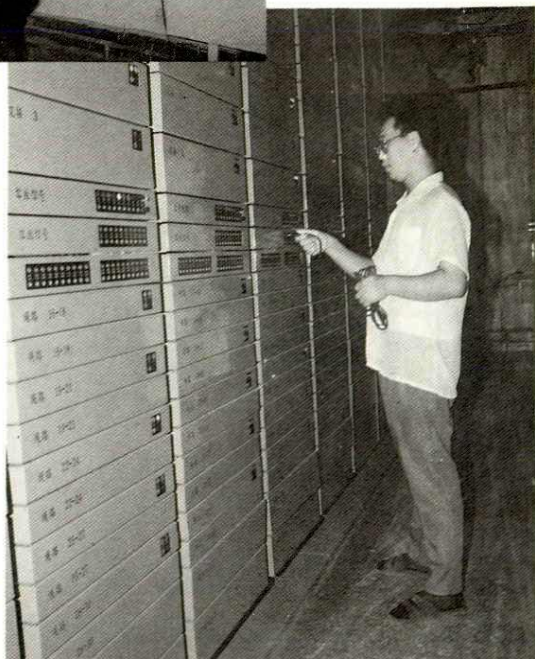
▼ 1989 年 9 月投入运行的市话 921 纵横制交换机
