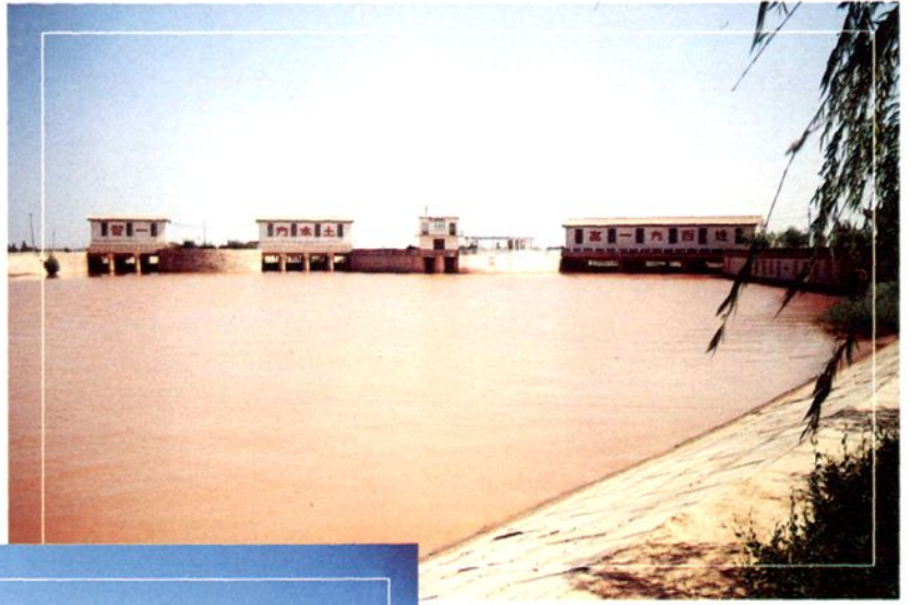
总干渠第二分水枢纽
