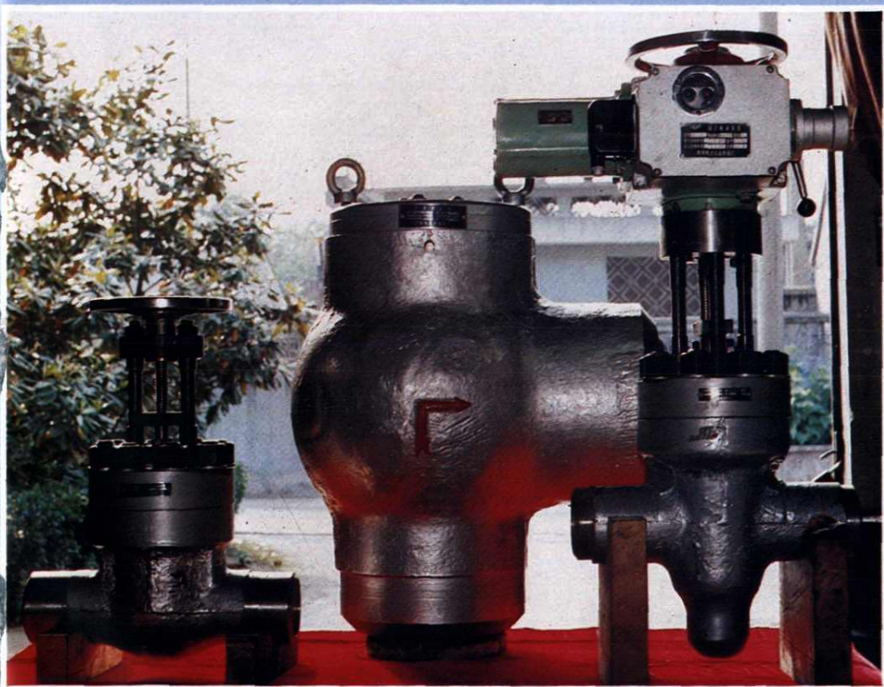
湖州发电厂引进先进技术制造的 (左起) J61Y25C 截止阀、H62Y25C 直角逆止阀、L961Y25C 再循环阀
