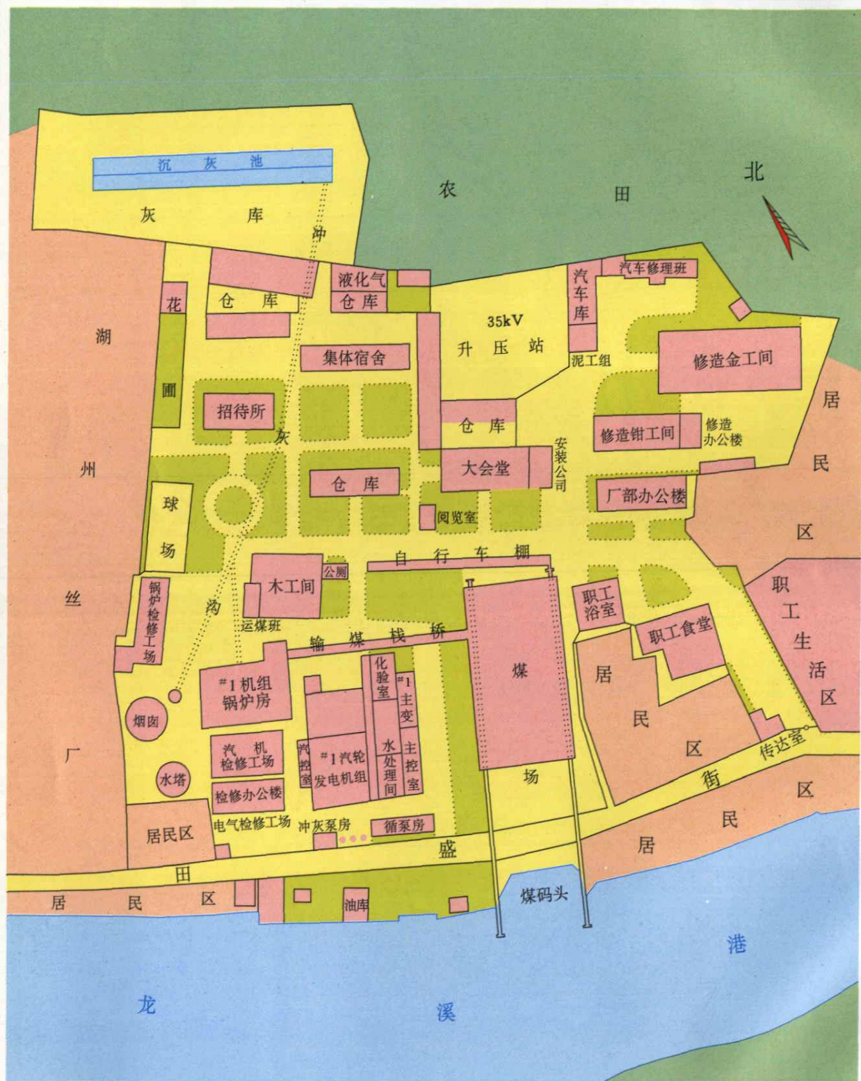
湖州发电厂厂区平面示意图
