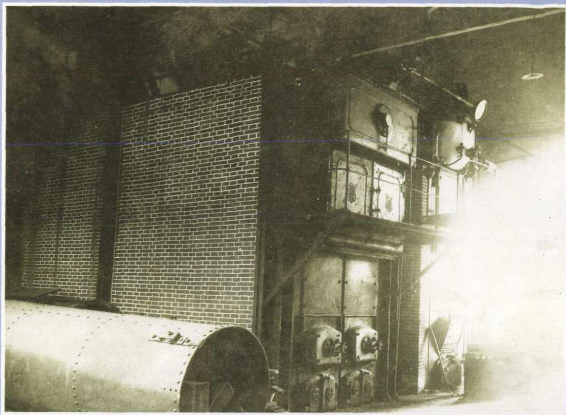
1914 年安装的蒸汽机锅炉
