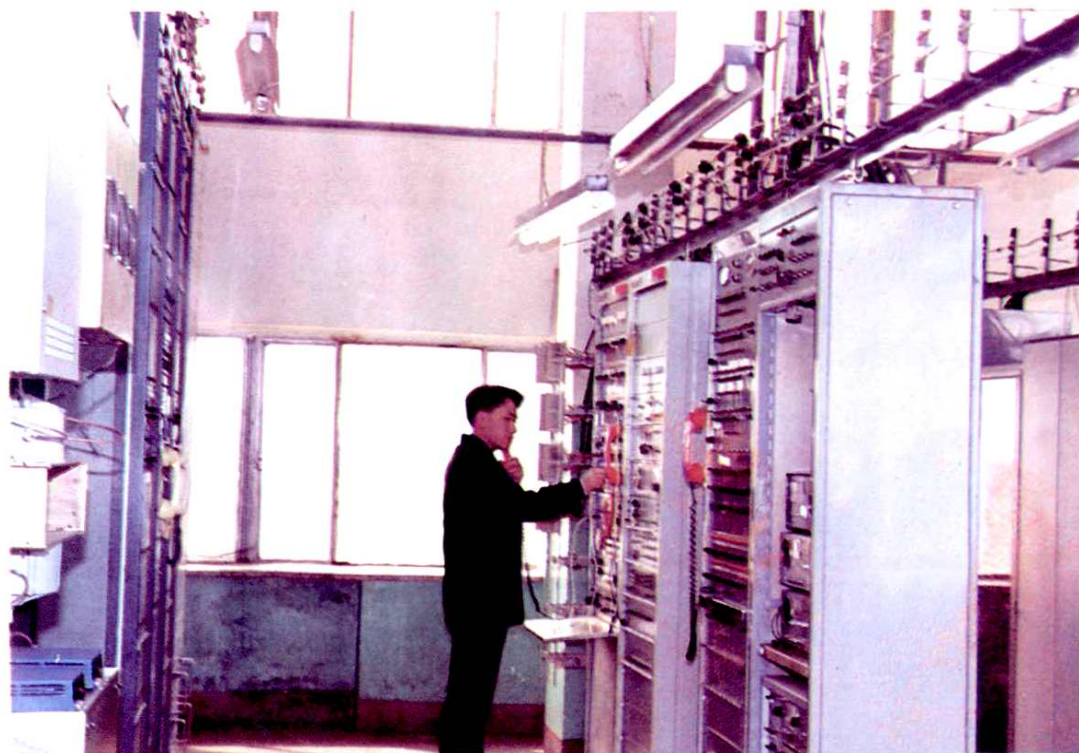
载波设备
