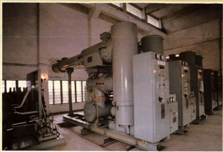
韶关电力工业局 110KV 河西变电站三菱 SFMT 断路器
