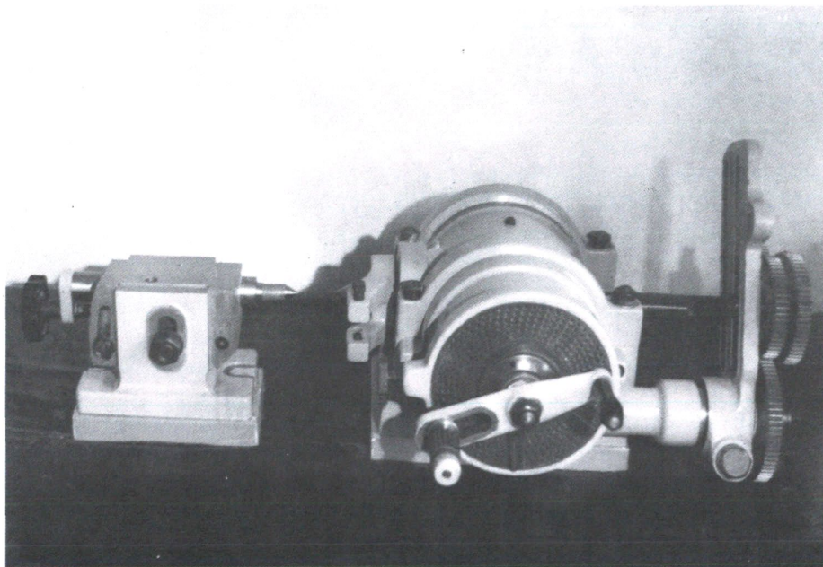
FW型万能分度头
