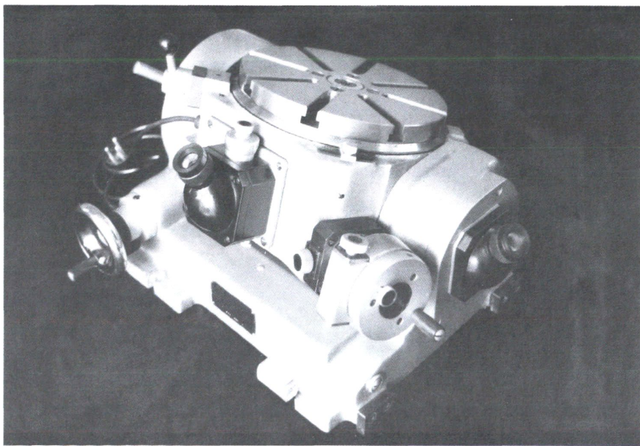
TGK可倾光学回转工作台
