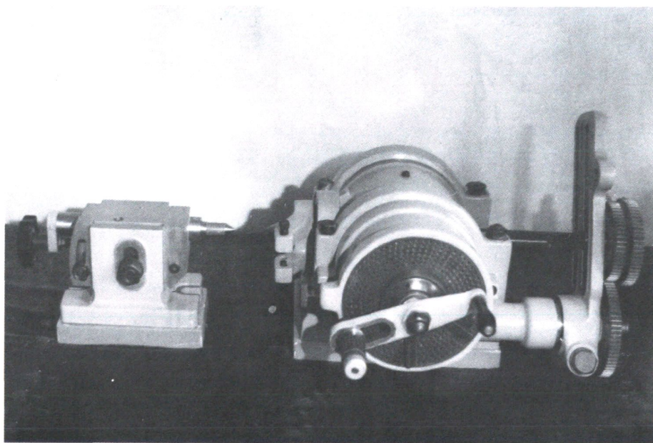
FW100、FW125、FW160型万能分度头
