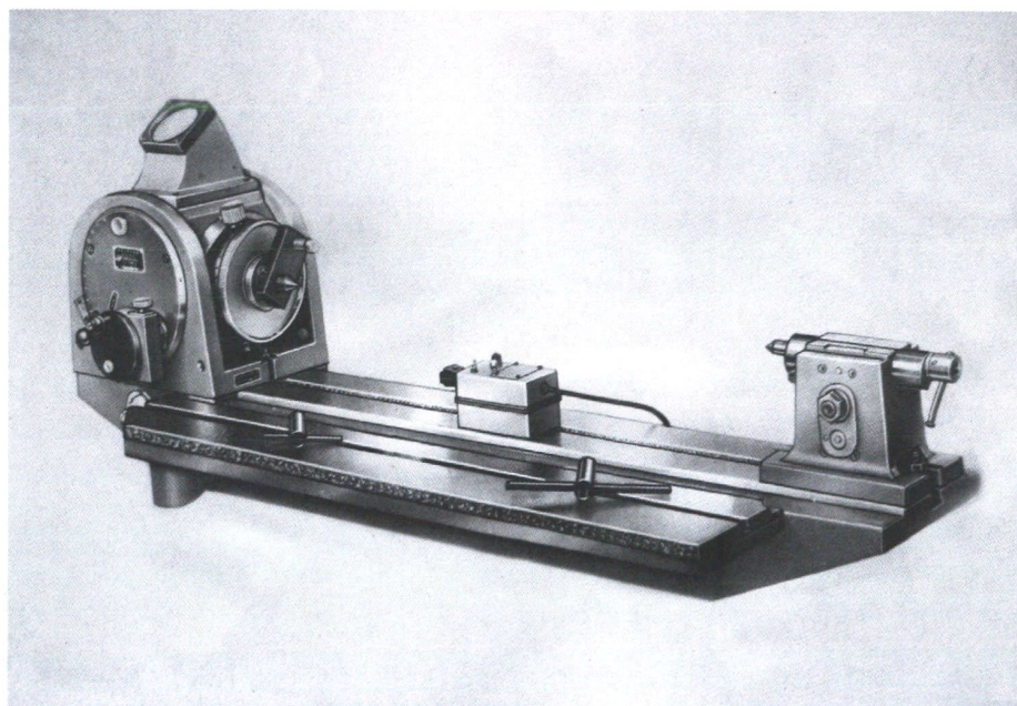
FP130A影屏光学分度头
