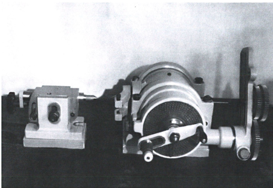
FW型万能分度头 (80、100、125、160)
