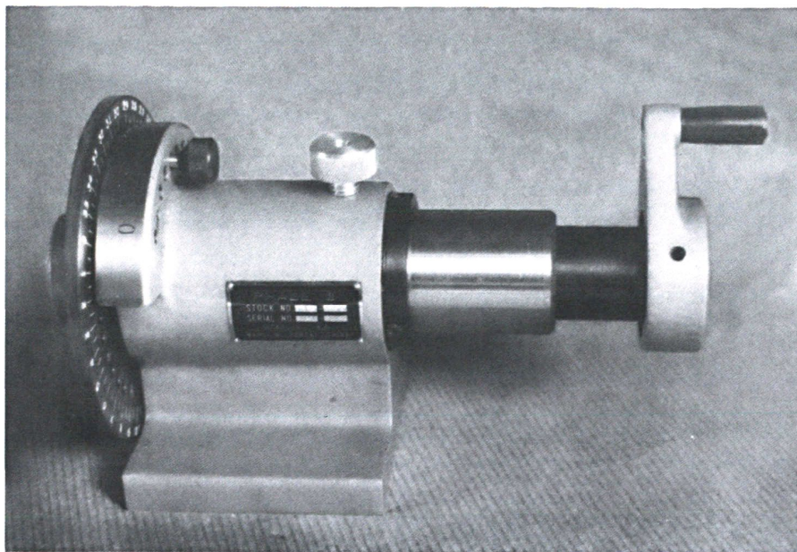
F1型5C旋转分度装置
