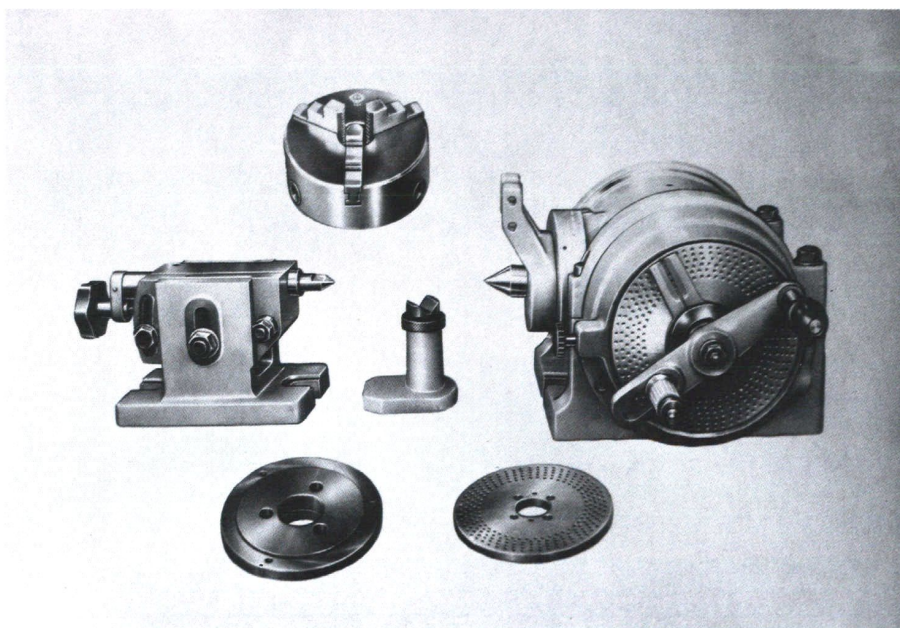
FB型分度头 (80、100、125、160)
