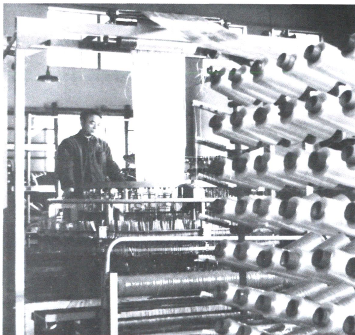
塑料圆筒编制机
