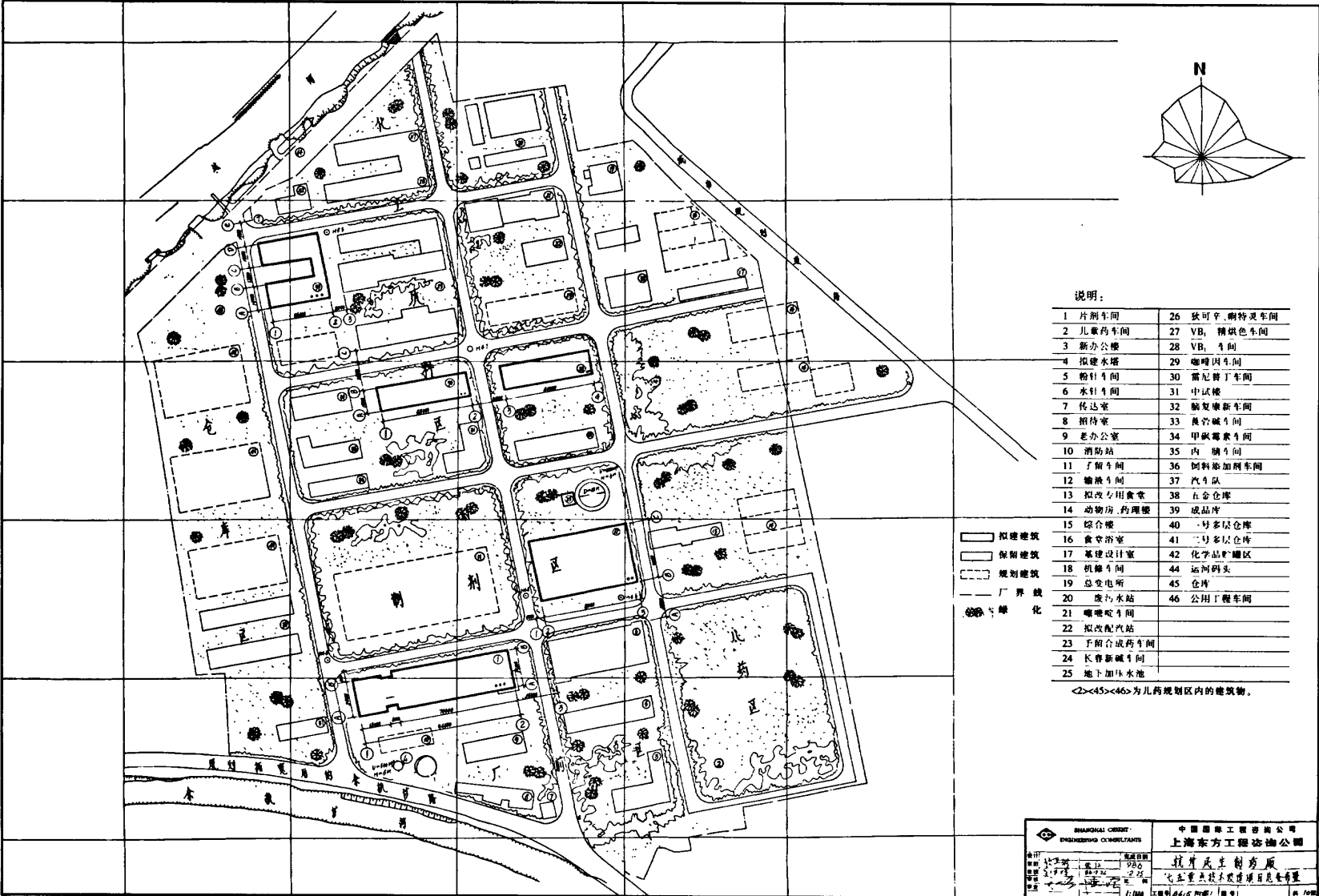
杭州民生药厂“七五”规划图
