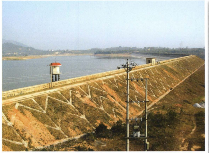
▶ 竹坝水库大坝全景图
