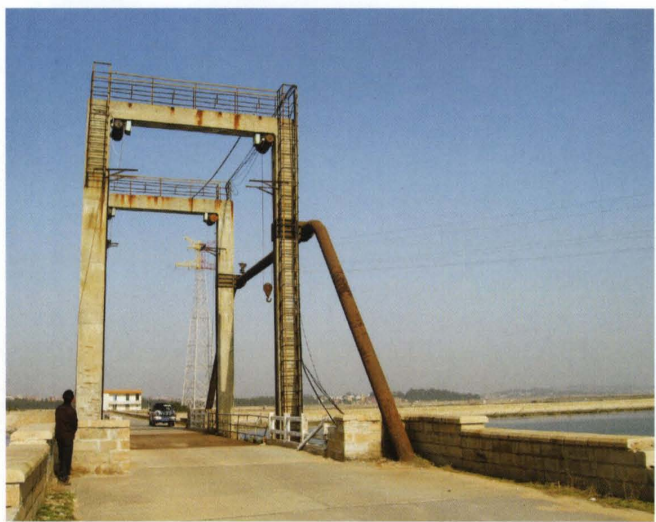
▼ 大嶼供水工程——大嶼海堤
