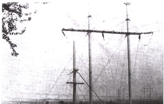
■1957年2月山东省第一条110千伏输电线路 神头发电厂至济南南郊变电站输电线路建 成投产。
