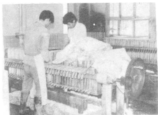
食品厂汤圆粉车间板框式过滤机一角
