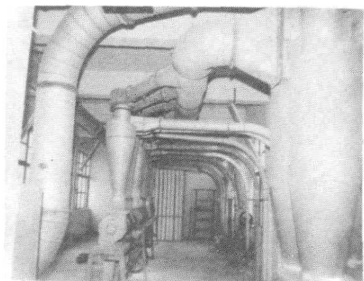
面粉厂风运设备一角
