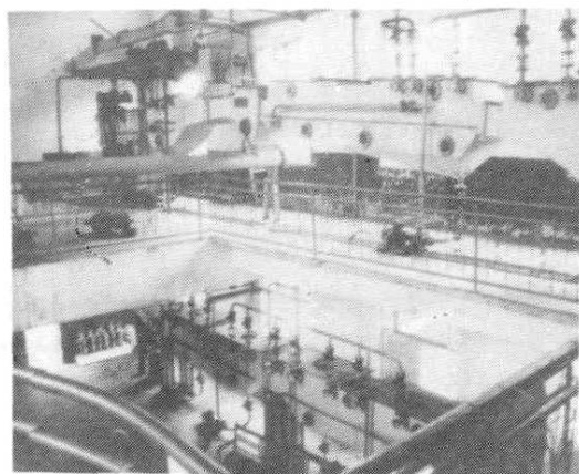
油厂浸出车间环形浸出器一角
