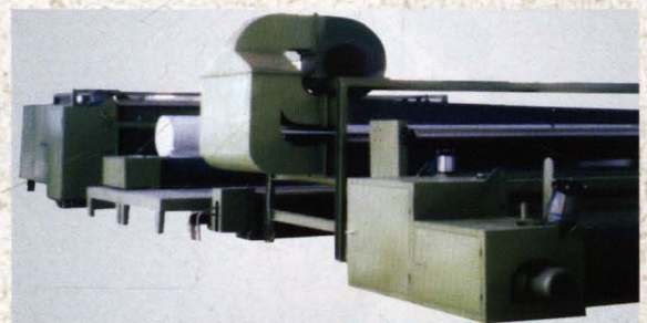
复合防渗土工膜复合生产线
