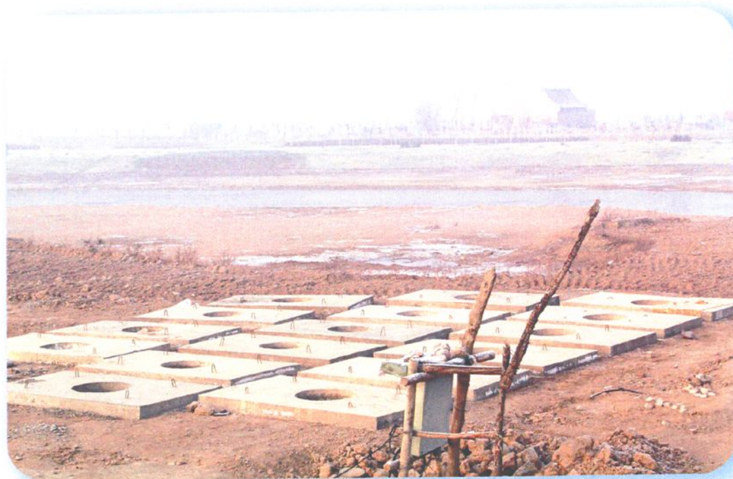
景观水道（来佛寺段）扩挖
