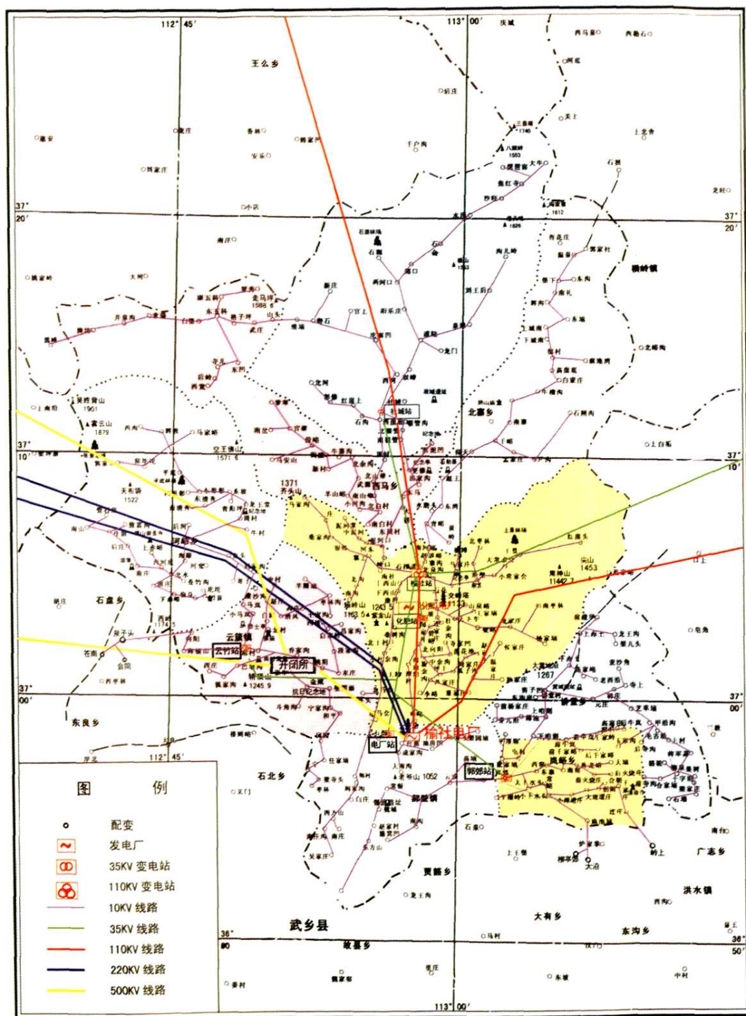
2004年榆社县输配电线路地理图
