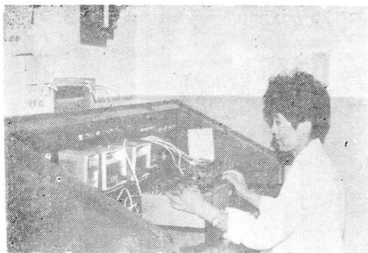
热工检定人员在进行二等标准热电偶检定
