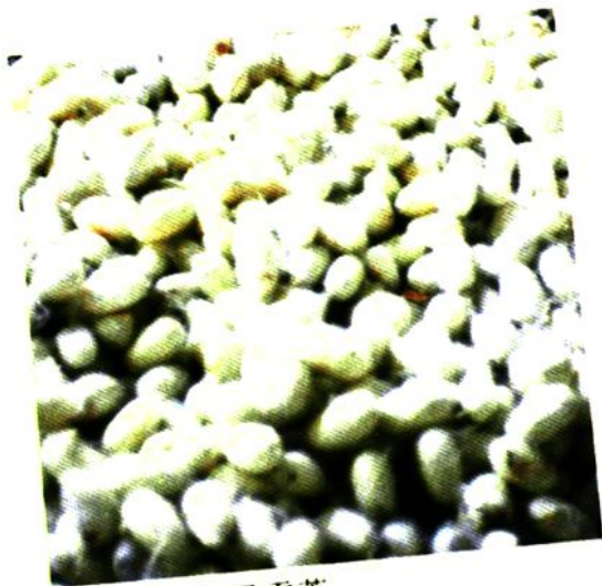
15. 桑蚕茧
