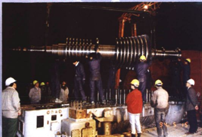
1994年5月15日，江苏射阳港发电有限责任公司 1号汽轮机转子吊装
