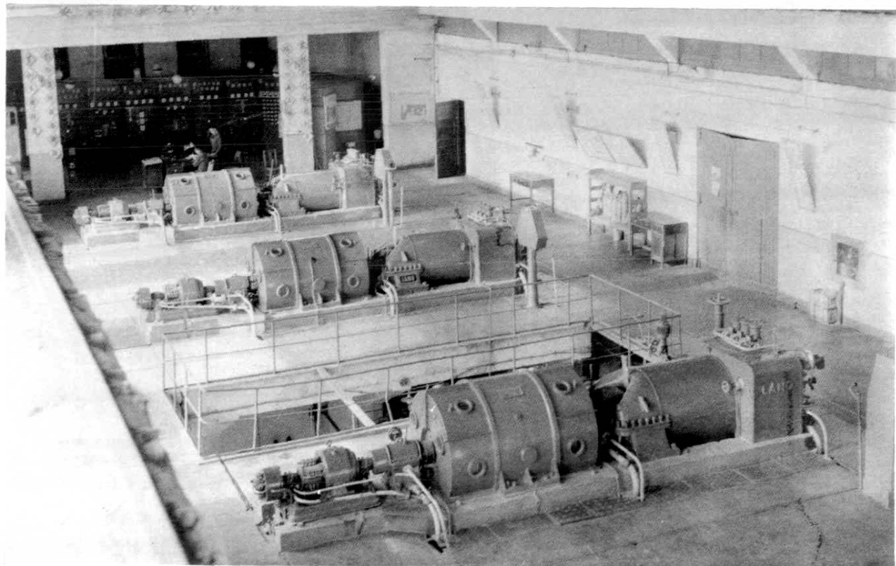
8 西宁发电厂4×1500千瓦汽轮发电机组
