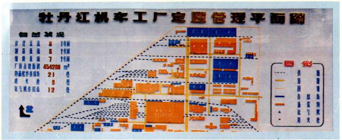
1989年工厂定置管理平面图
