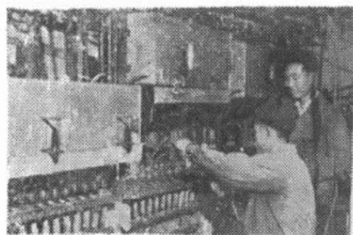
灯泡封排设备
