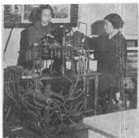
灯泡芯柱机
