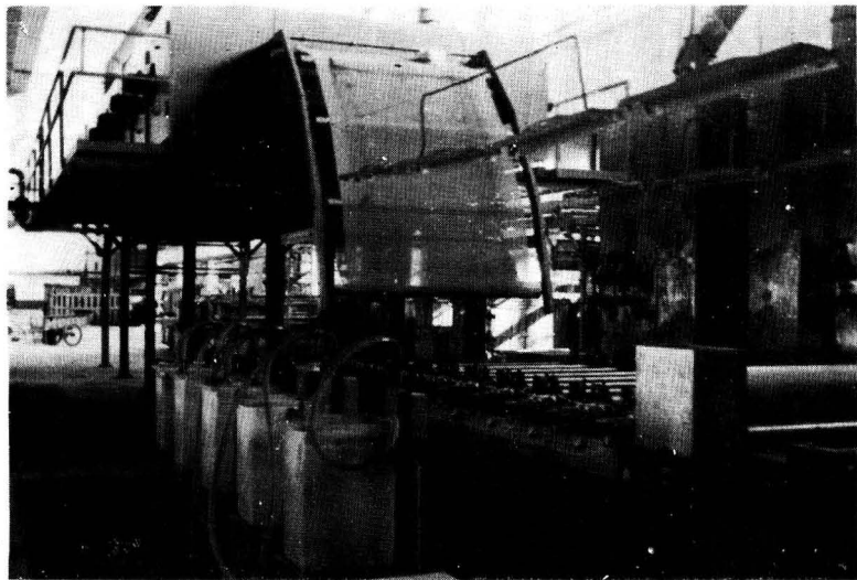
园网印花机
