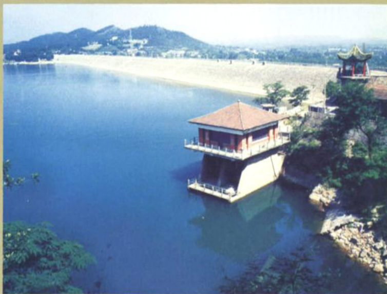
② 输水洞进口
