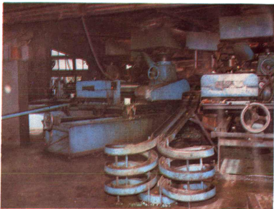
1、沈阳玻璃厂玻璃纤维球生产线
