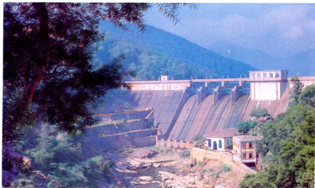
△1958年建成的东张水库大坝,是省建的第一座砼坝,坝高38米。
