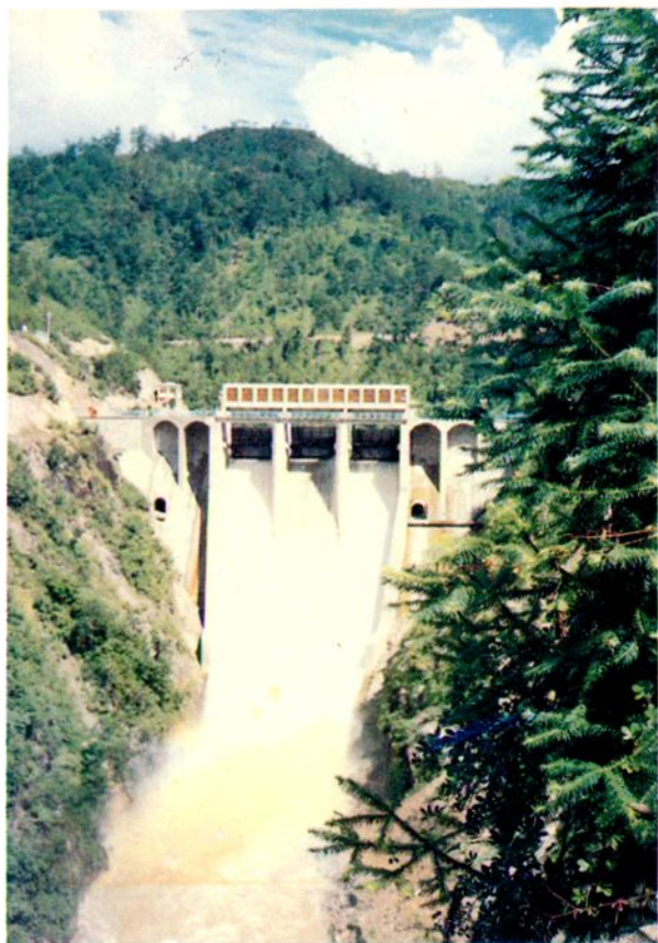
△我国第一座碾压砼坝
