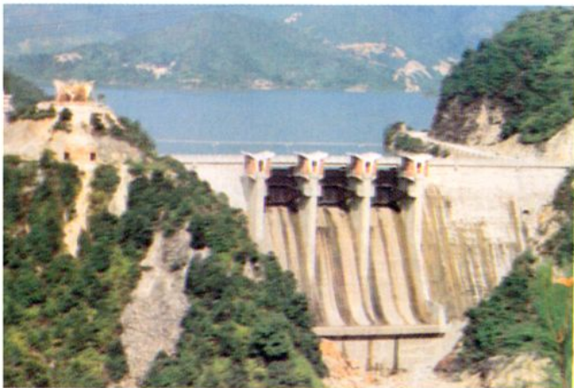
龙门滩碾压砼坝,高 57.5m,长 189m,1989 年建
