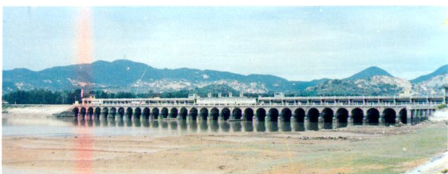
洛阳桥闸 32 孔长 205m, 1974 年建, 是山美水库第二分水枢纽。
