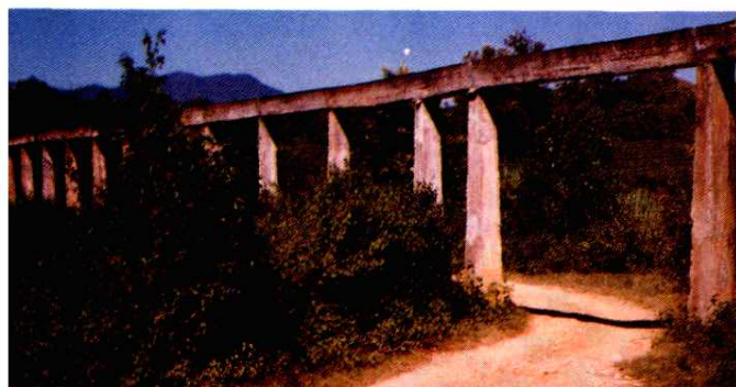
引水长渡槽（30 米）
