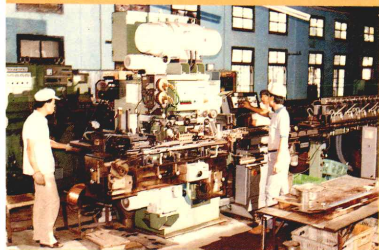
↓ 从国外引进的高频焊接空罐生产线
