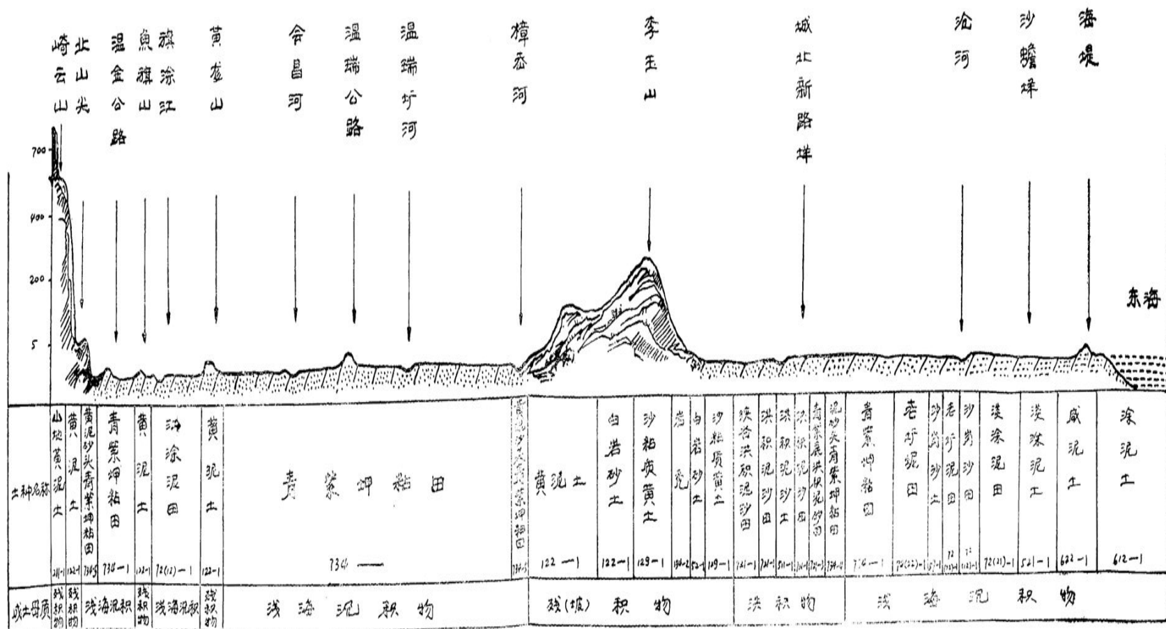
沙蟾乡、仰义乡河岱山断面图
