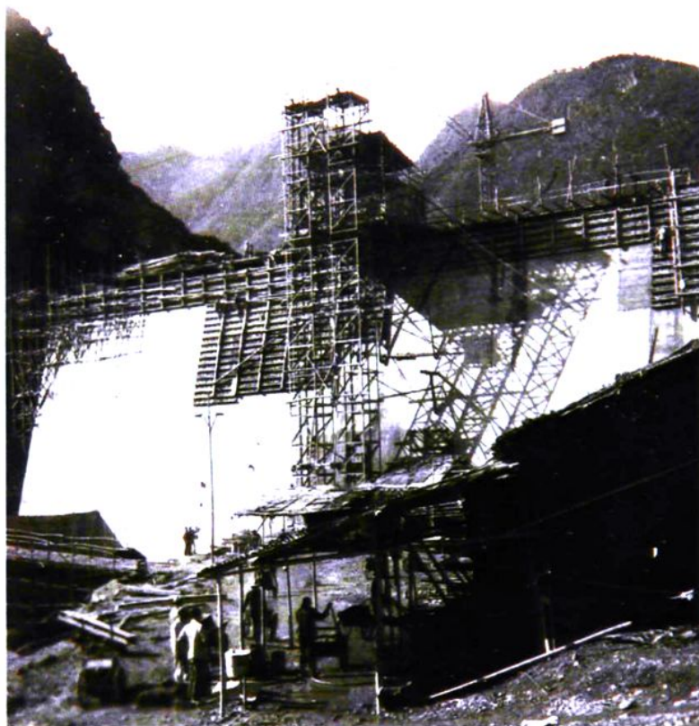
新昌长诏水库施工
