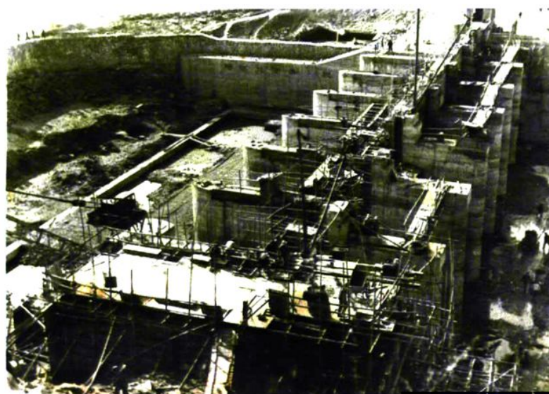
海盐长山闸施工
