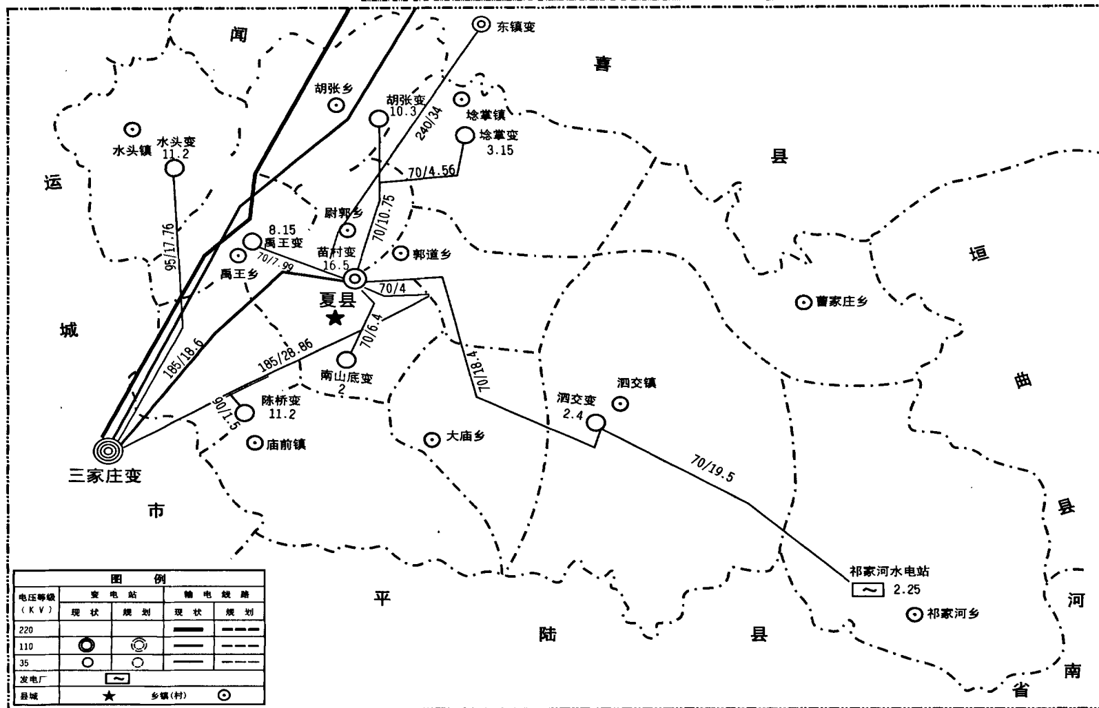
【夏县电力系统地理接线示意图】
