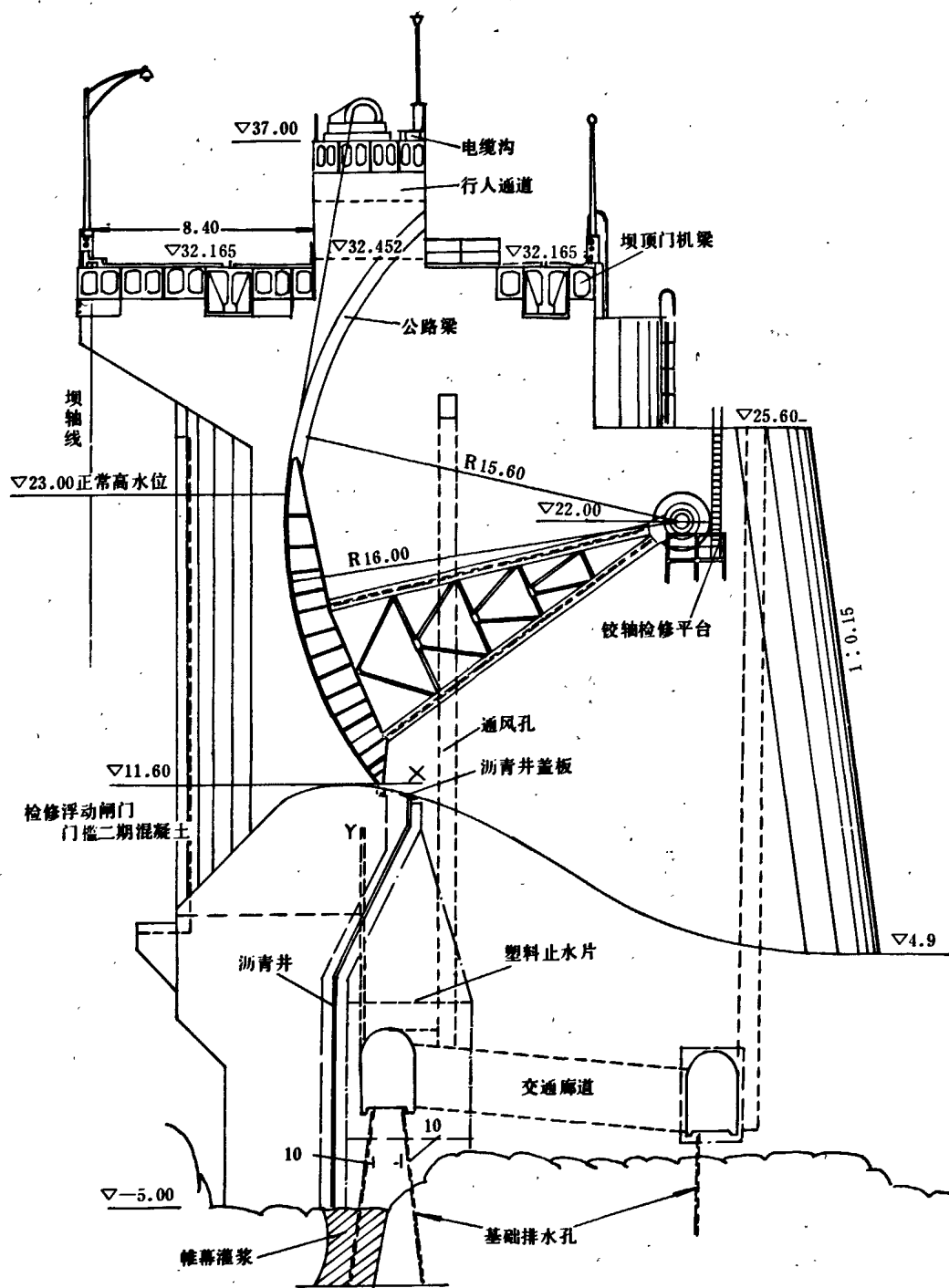
溢坝标准剖面图
