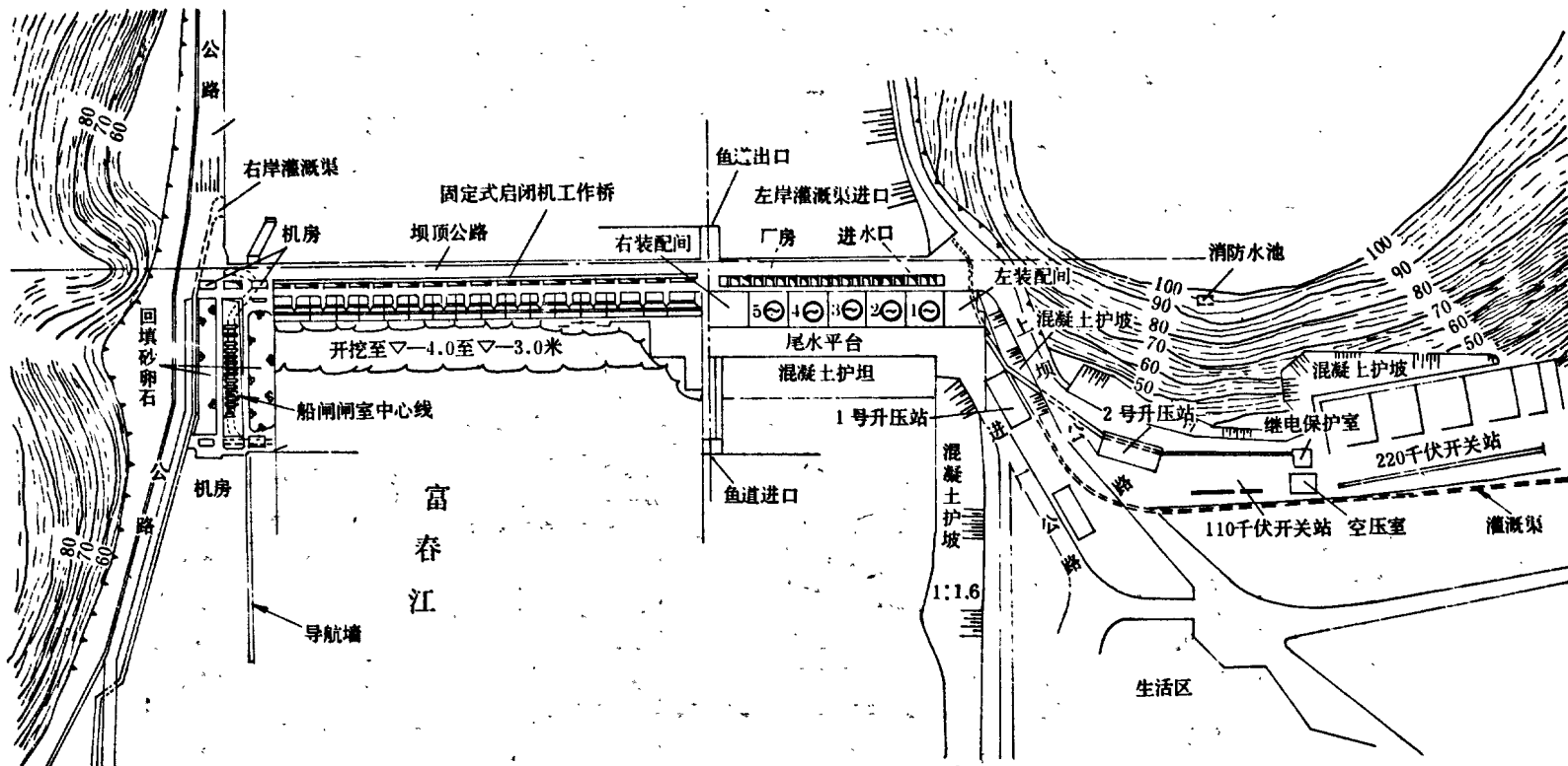
富春江水电站水力枢纽总体布置图
