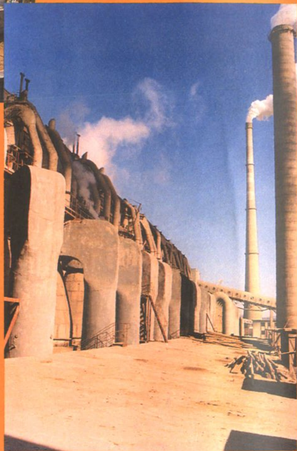
辽宁发电厂麻石水膜除尘装置
