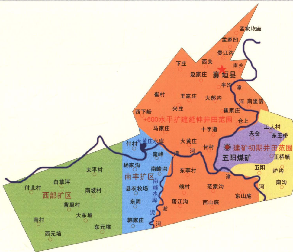
潞安矿区五阳煤矿平面图
