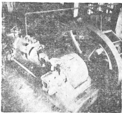
原郎溪县明星电灯公司的德国茅士尔厂制造的 40 马力卧式柴油机
