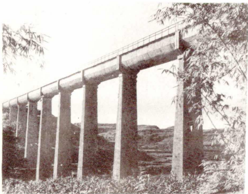
夏家坝渡槽
