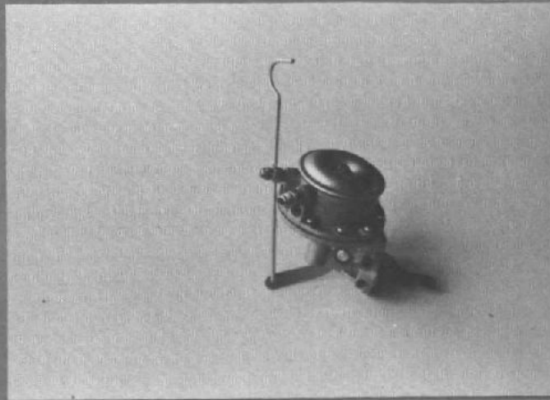
▲ EQB601 型汽油泵
