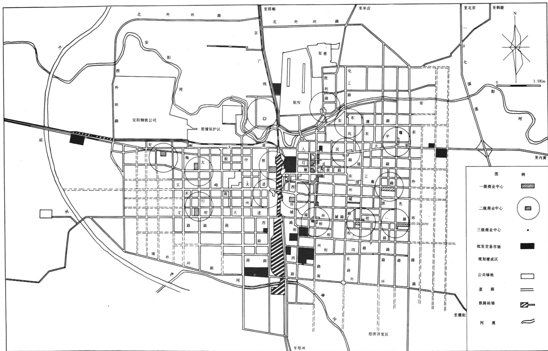
图 2-9 安阳市区商品市场体系总体规划图
