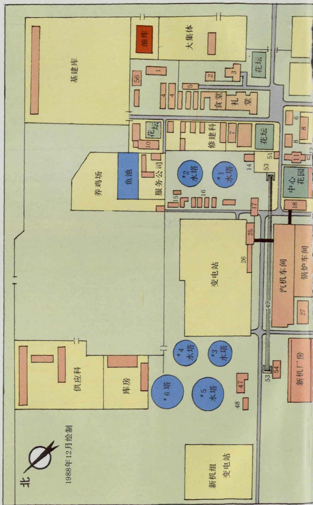
包头第二热电厂厂区平面图
