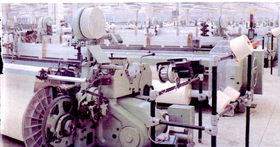
瑞士苏尔 寿片梭织机
