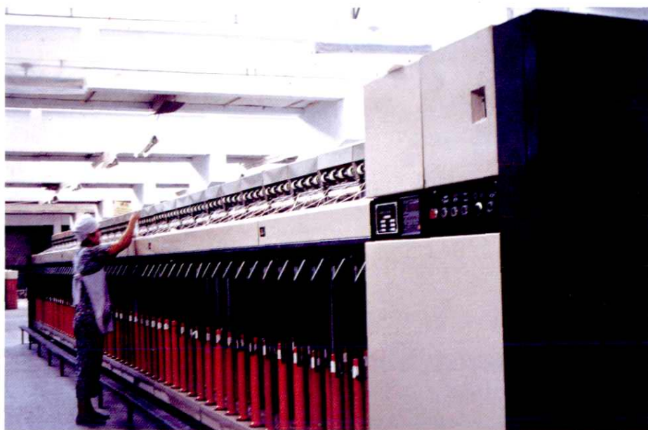
FA421型粗纱机
