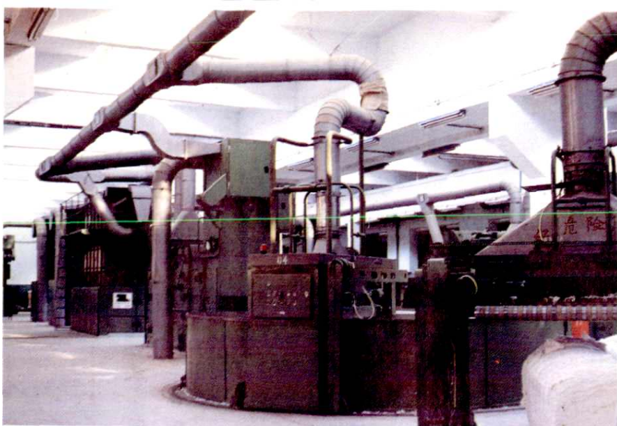
刘忠恕 1970 年发明的 A002A 型 单轨环行抓棉机, 1978 年获国家 科委四等发明奖
