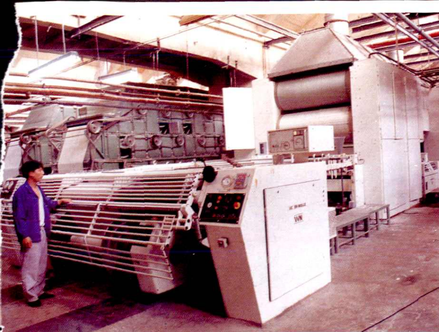
德国祖克浆纱机
