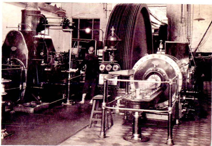
从建厂到1958年，全厂生产动力源——800匹马力蒸汽引擎
