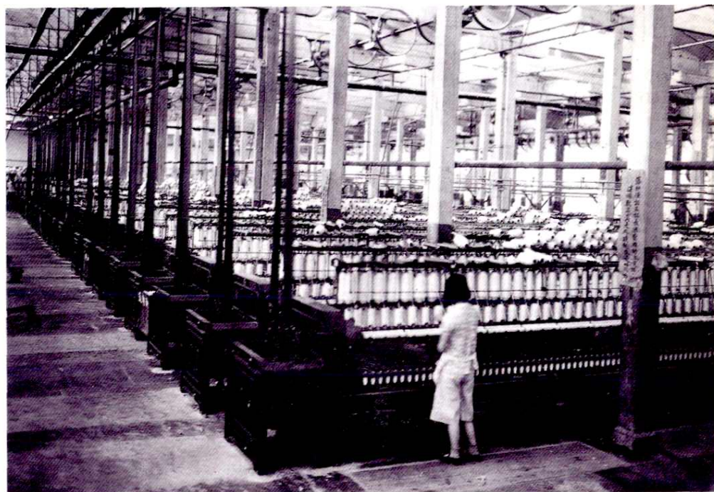
解放初期天轴皮带 传动细纱机工作情形
