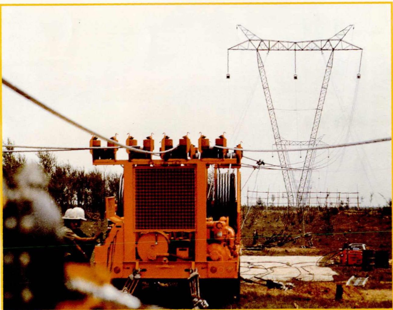
公司承建施工的太原至神头 500 千伏线路工程,施工人员正在张力放线
