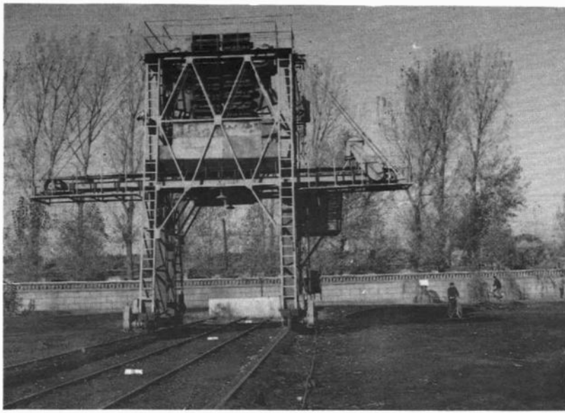
朝阳市燃料公司 煤场的龙门吊作业
