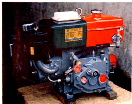
国优产品 R175A 柴油机
