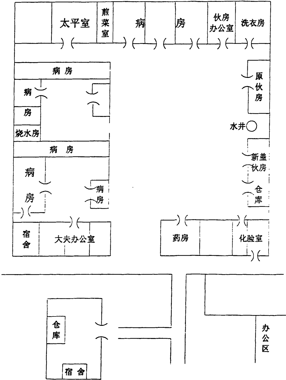
桃园病房草图
