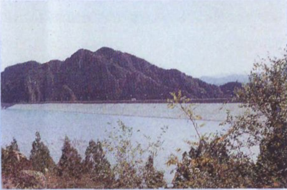
1959~1960年，基础总队承建的北京密云水库白河主坝防渗墙，是国内第一道槽孔型防渗墙
