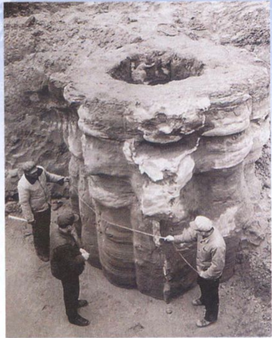
20世纪70年代，四川龚嘴水电站高喷围井试验开挖后直观图
