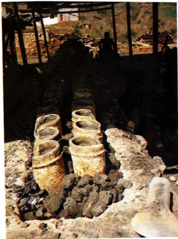
马 槽 炉
