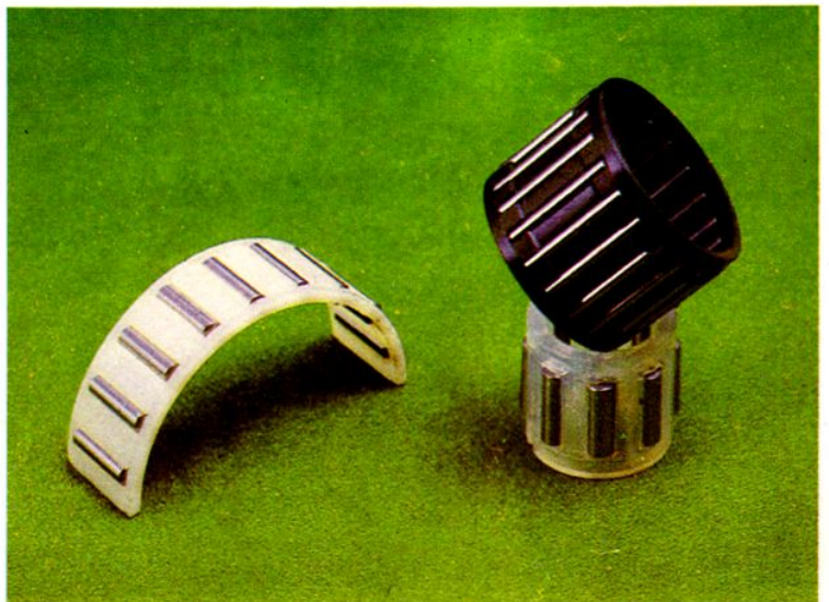
紡織機械專用滾針軸承
