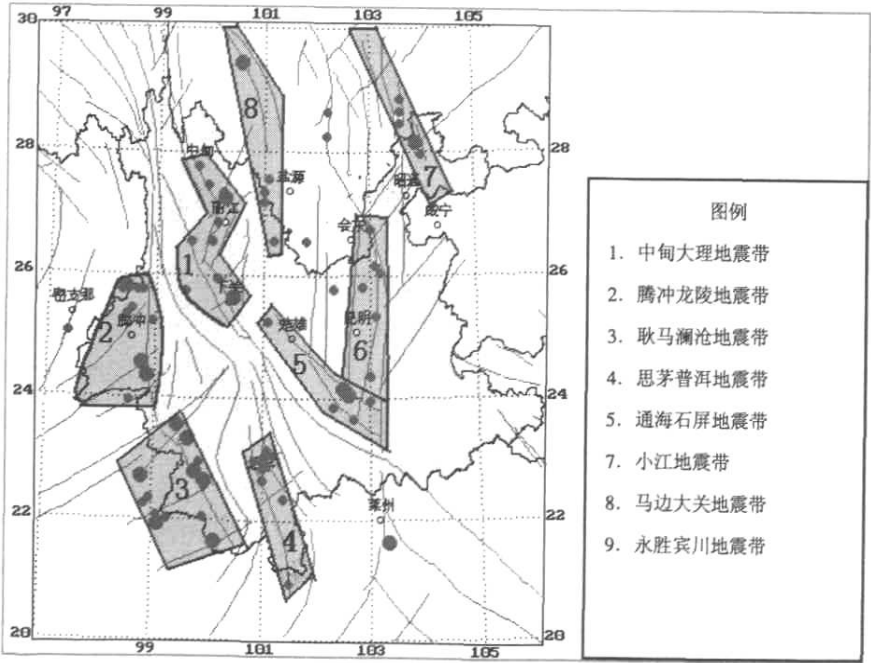
图 1.1.2 云南地区地震带（区）分布图
