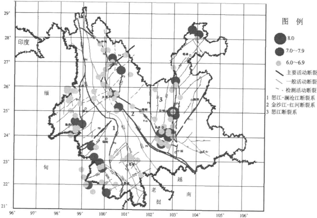
图 1.1.1 云南省 6 级以上地震分布及地质构造简图
