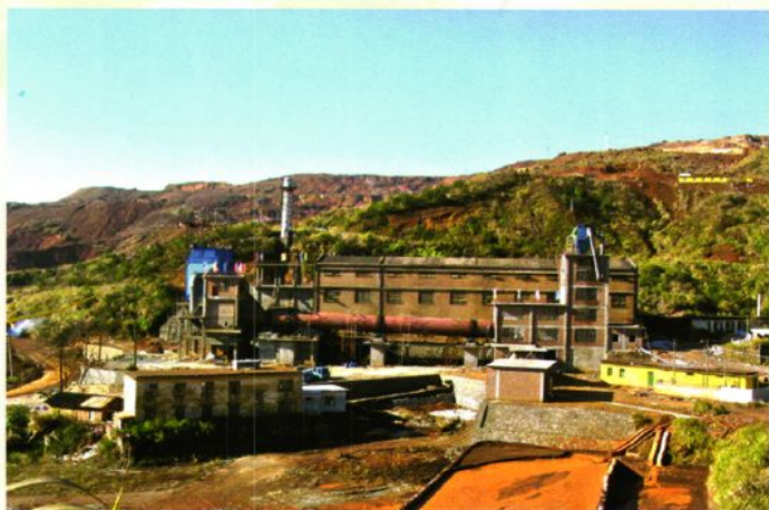
磁化焙烧厂
