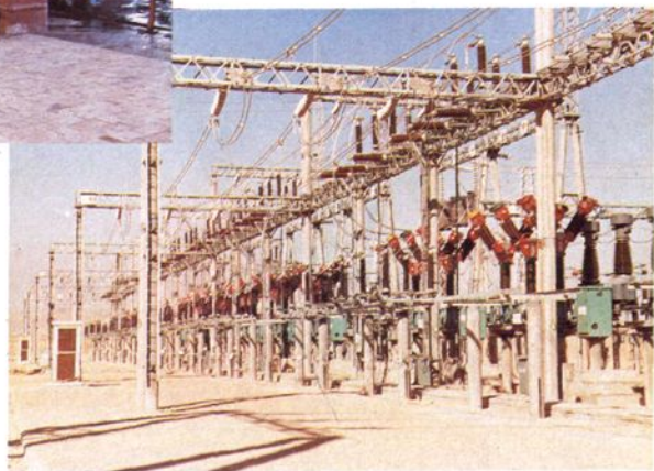
▼即将投入运行的海永线330千伏变电站
