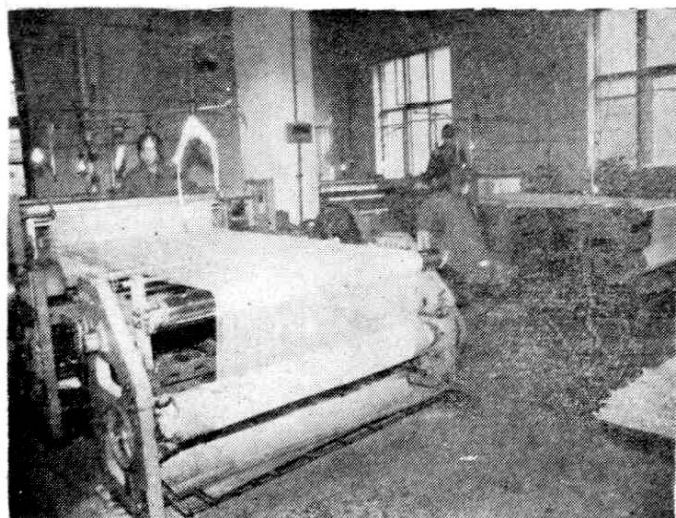
丝织车间（二）
