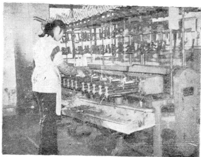
丝织车间（一）
